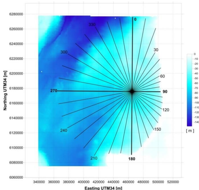
IV.1 paveikslas. Azimutinių profilių schema su tyrimų zonos batimetrija. Jūros gylis metrų. Koordinatės UTM34 zonoje. Batimetrinių duomenų šaltinis: BSHC duomenų bazė (data.bshc.pro).
