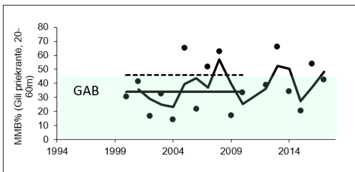
5 paveikslas. CB% ir MMB% kaitos tendencijos (2 m slenkančių vidurkių kreivė), vidutinė daugiametė reikšmė 2000-2010 (juoda ištiesinė linija), GAB sritis pažymėta žaliai pagal 95 % pasikliautinių intervalų (punktyrinė linija) ribą. Paliginimo patogumui, zonų pavadinimai (gili priekrantė, sekli priekrantė) pateikti, tokie, kokie buvo JSPD pradiniam (iki 2011 m.) vertinimo ciklo, atitinkamai: Zona BAL_LT-AA-03 ir Zona BAL_LT-AA-01.
