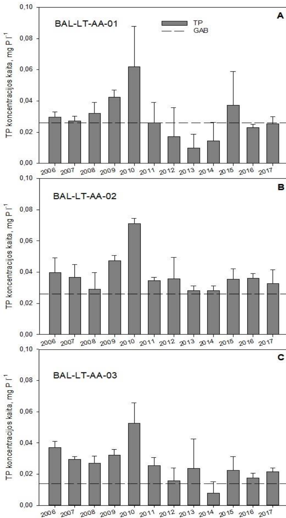
3.3.1.3 paveikslas. Vidutinė bendro fosforo (TP) koncentracija priekrantės (A), tarpiniuose (B), teritorinės ir atviros jūros (C) vandenyse 2006–2017 metais. A, B – vasaros (06-09 mėn.), C – metinė. Punktyrinė linija žymi GAB reikšmę.
