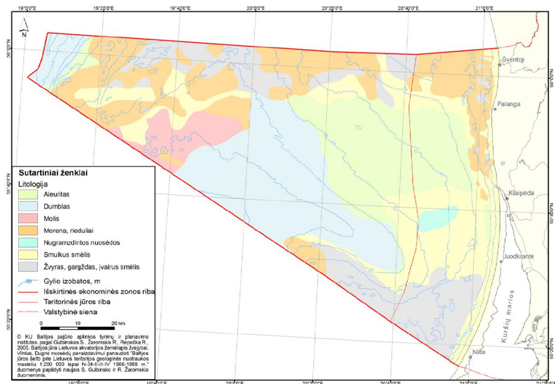
2.3.1 paveikslas. Baltijos jūros Lietuvos akvatorijos dugno reljefas (pagal Gelumbauskaitę, 1998) ir dugno nuosėdų tipų paplitimas (Žaromskis ir kt., 2005).
