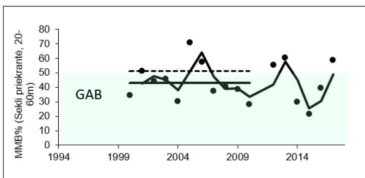
6 paveikslas. MMB% kaitos tendencijos (2 m slenkančių vidurkių kreivė), vidutinė daugiametė reikšmė 2000-2010 (juoda ištiesinė linija), GAB sritis pažymėta žaliai pagal 95 % pasikliautinių intervalų (punktyrinė linija) ribą.
