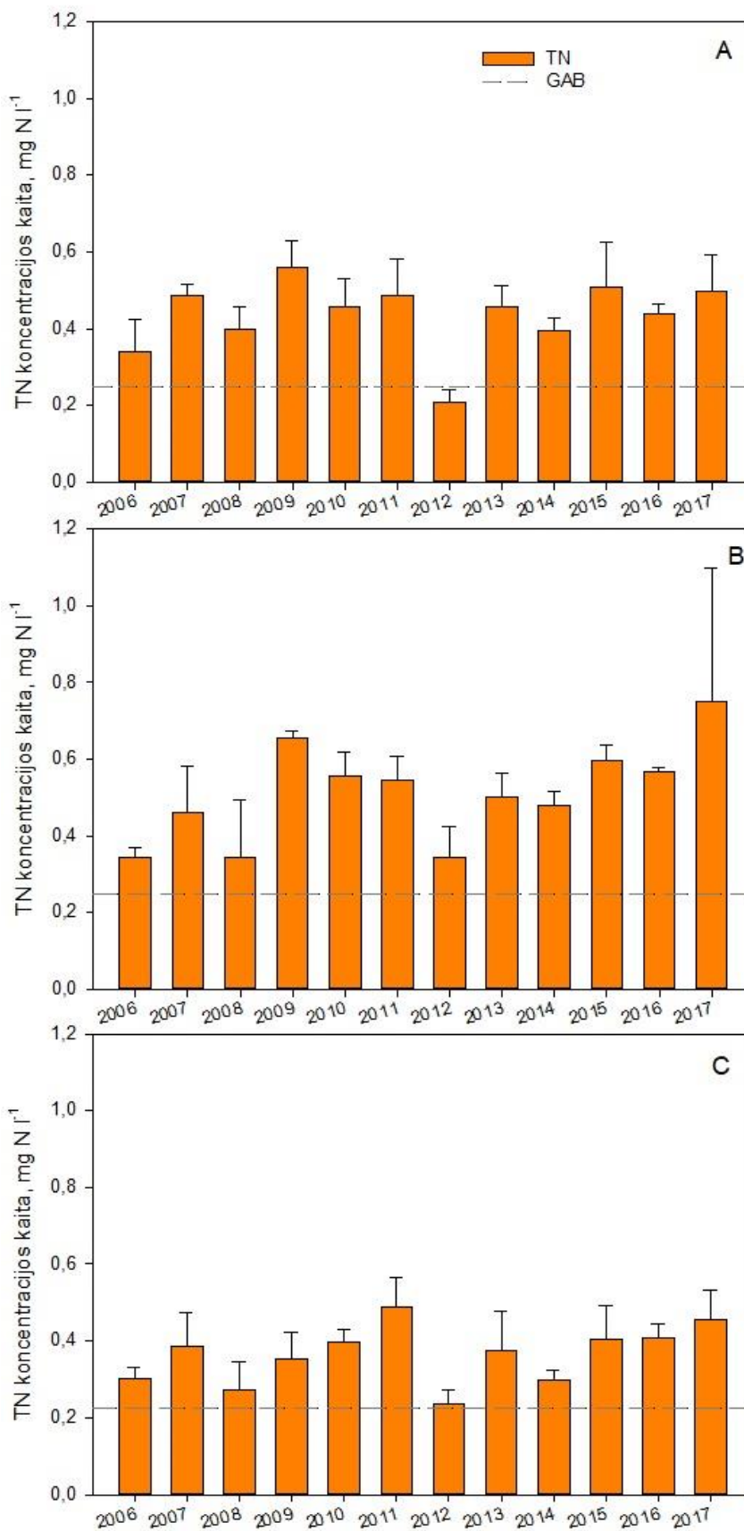
3.3.1.1 paveikslas. Vidutinė bendro azoto (TN) koncentracija priekrantės (A), tarpiniuose (B), teritorinės ir atviros jūros (C) vandenyse 2006–2017 metais. A, B – vasaros (06-09 mėn.), C – metinė. Punktyrinė linija žymi GAB reikšmę.
