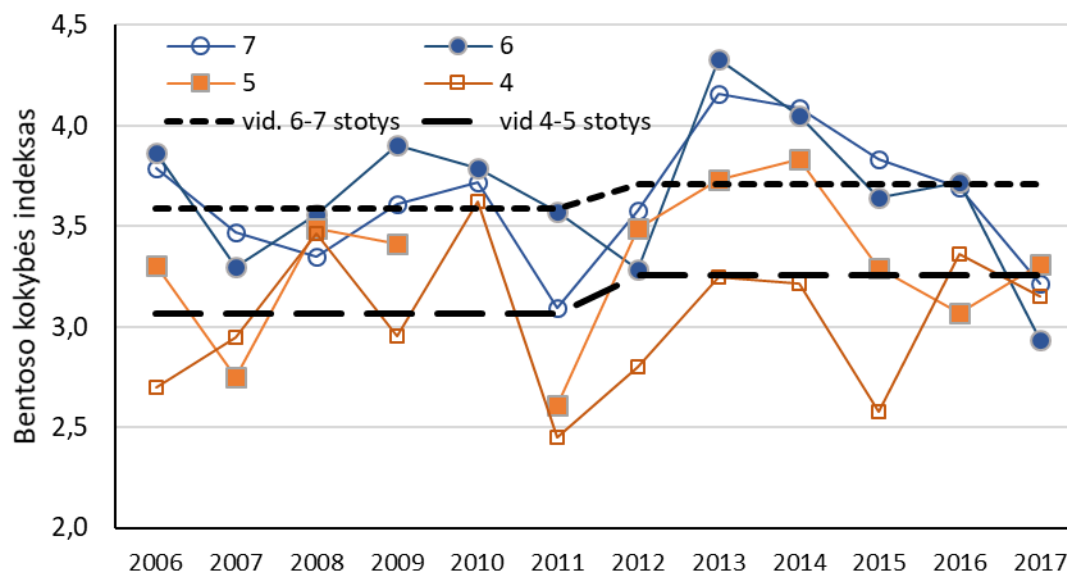
3.3.1.15 paveikslas. Dugno makrofaunos būklė 2006-2017 m. pagal BKI priekrantės vandenyse (4, 5, 6 ir 7 stebėsenos stotys). GAB vertė 3,2.
