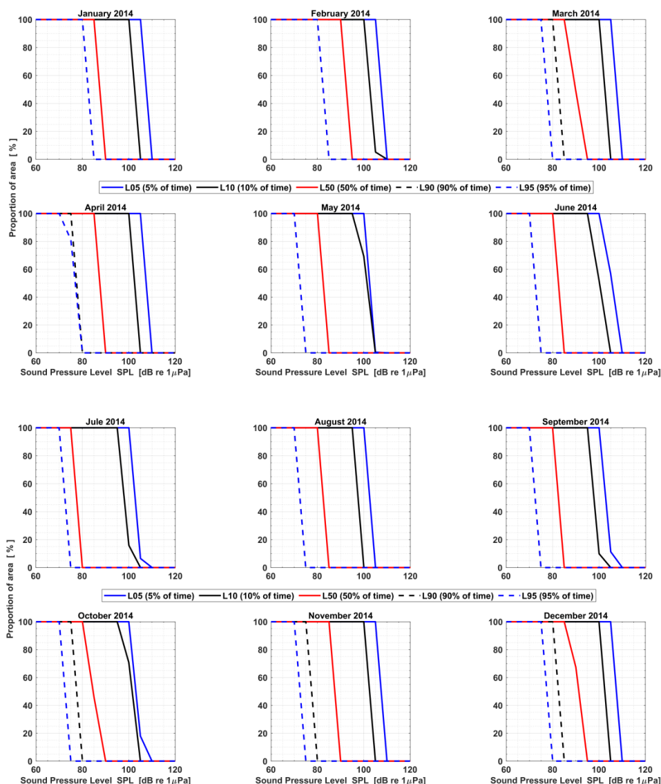
3.3.5.4 pav. Garso slėgio dažnio lygis skirtingais mėnesiais (remainis 2014 m BIAS projekto duomenimis).
