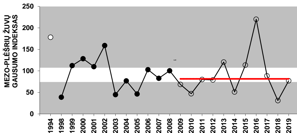
4.1.1.32 paveikslas. Kertinių Baltijos jūros priekrantės žuvų funkcinių grupių gausumo (Mezo-plėšrių žuvų gausumas) indeksas ir jo kaita pagal žuvų monitoringo duomenis Baltijos jūros priekrantėje (● – referentiniai duomenys, ○ – vertinamas periodas) 1994-2019 m. (gera aplinkos būklė – šviesi zona, raudona linija – vertinamo periodo metinių medianų mediana, indikuojanti aplinkos būklę 2009-2019 metais).
