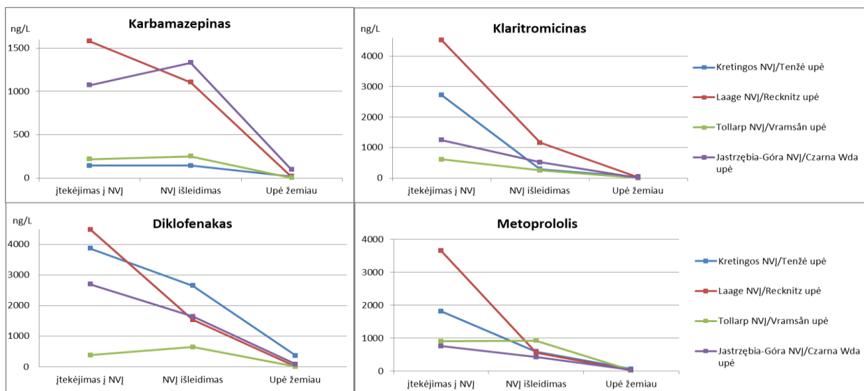
3.3.2.5 paveikslas. Vidutinės farmacinių medžiagų koncentracijos nuotekose ir upių vandenyje žemiau nuotekų valyklų
