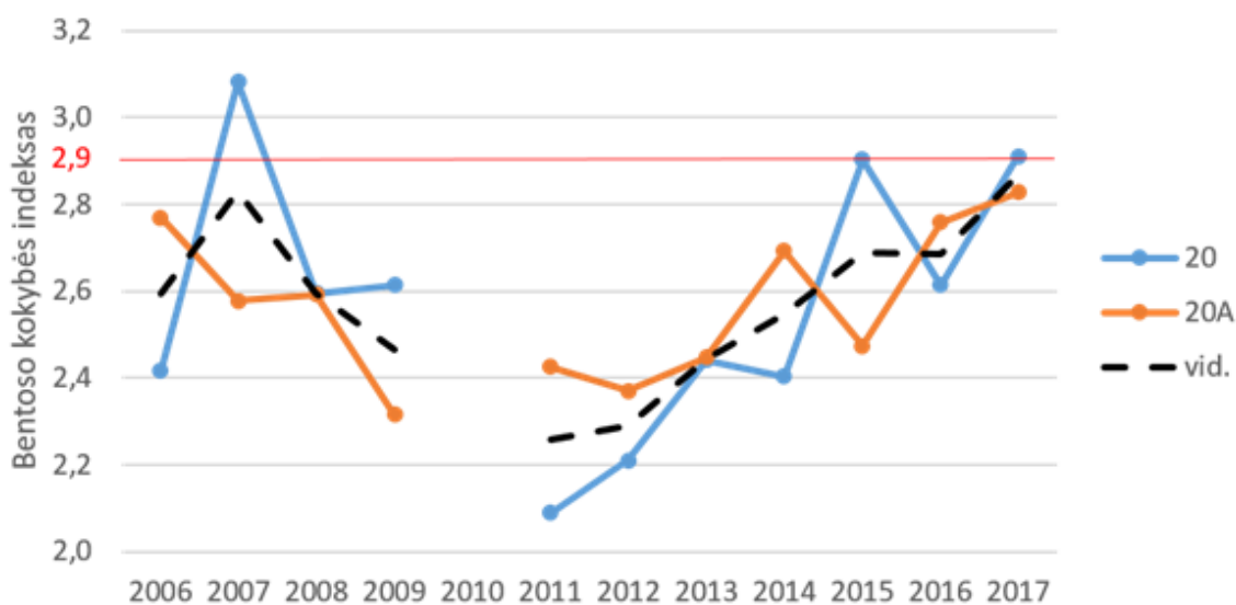
3.3.1.17 paveikslas. Dugno makrofaunos būklė dampingo rajono stotyse (20 ir 20A) 2006-2017 m. laikotarpiu.
